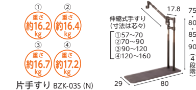
片手すり BZK-03S (N)
