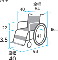
ノーパンクタイヤ
