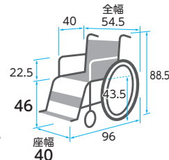
ノーバンクタイヤ
